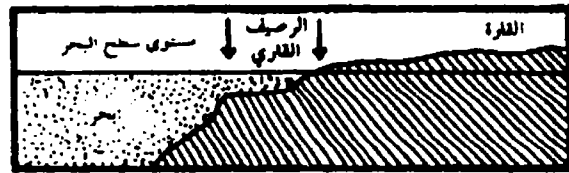
الرصيف القاري يستقبل بلايين الأطنان من الرواسب القارية والبحرية...
